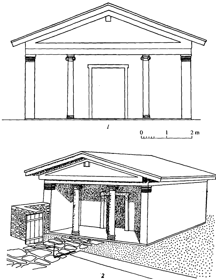
Рис. 3. 1–2 – реконструкция храма Юпитера Долихена на территории Балаклавы по Т. Сарновскому и О.Я. Савеле
