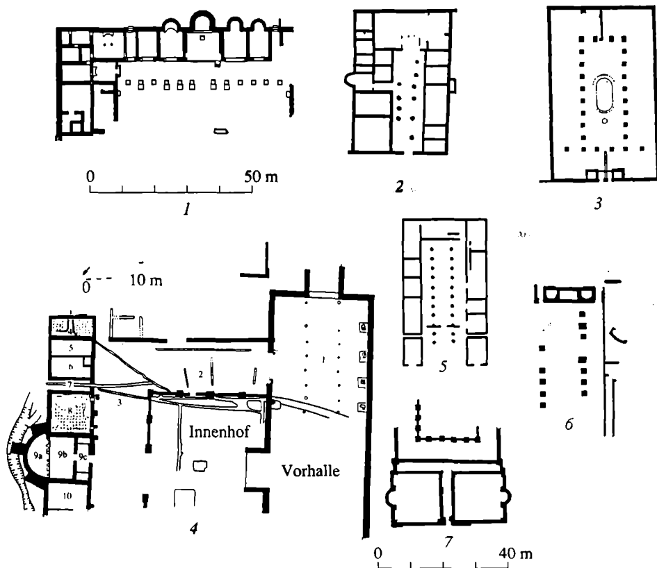
Рис. 5. Схематические планы из раскопок пунктов дислокации римских войск по Н. v. Petrikovits and R. Fellmann. 1 – Ламбесис, 2 – Карнунт, 3 – Новезиум, 4 – Аален, 5 – Инчтатхил, 6 – Церлеон, 7 – Ветера
