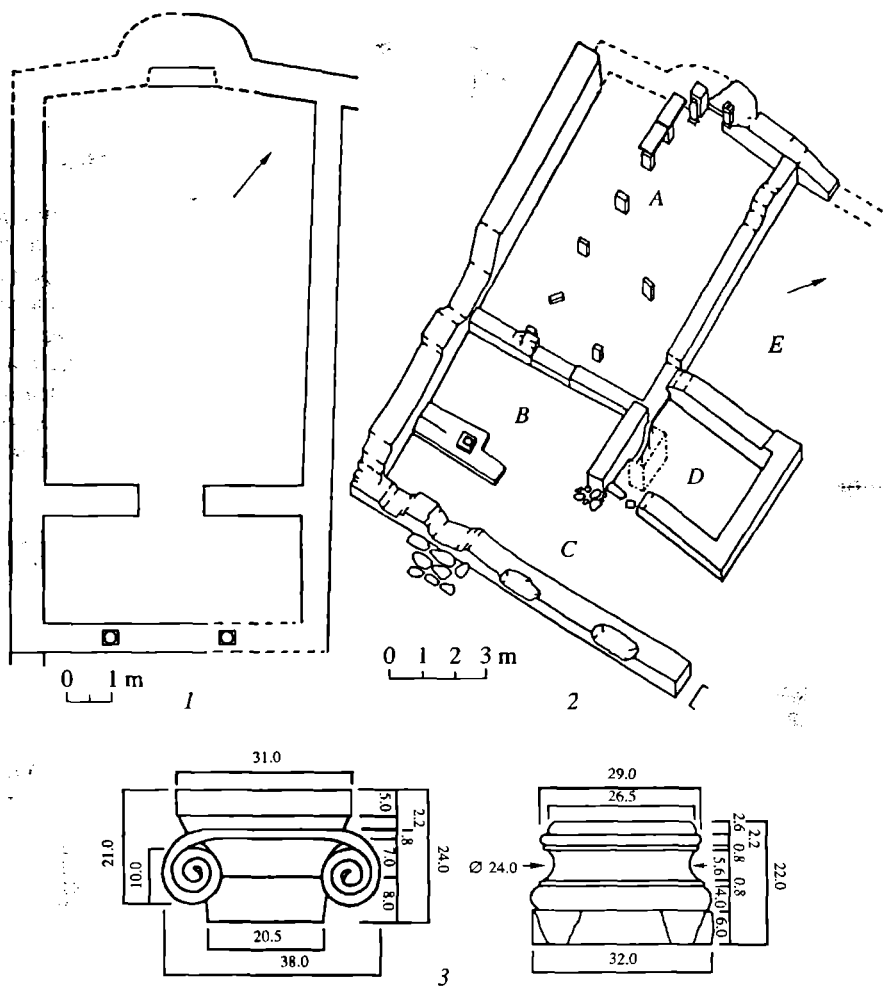
Рис. 4. 1 – план, 2 – аксиометрическое изображение и 3 – архитектурные детали из раскопок на территории Балаклавы по Т. Сарновскому и О.Я. Савеле
