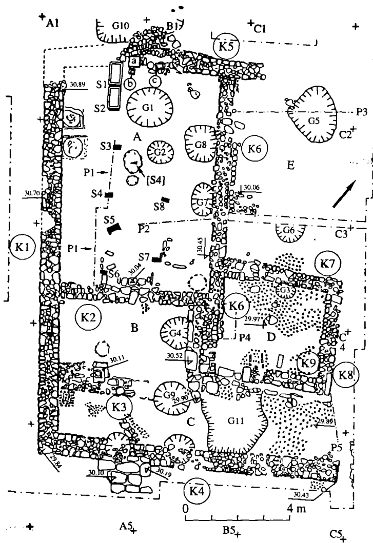
Рис. 1. План строительных остатков, раскопанных на территории Балаклавы в 1996–1997 гг. по Т. Сарновскому и О.Я. Савеле
